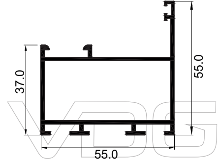
KK-102 Kanat 1,000 kg/m
