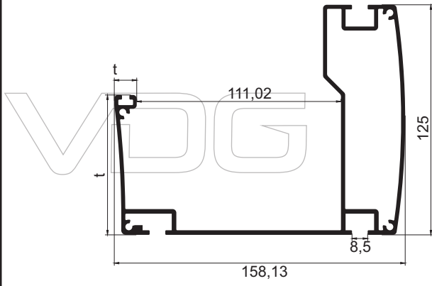
P-106 Orta Seri Oluk 3,916 kg/m
