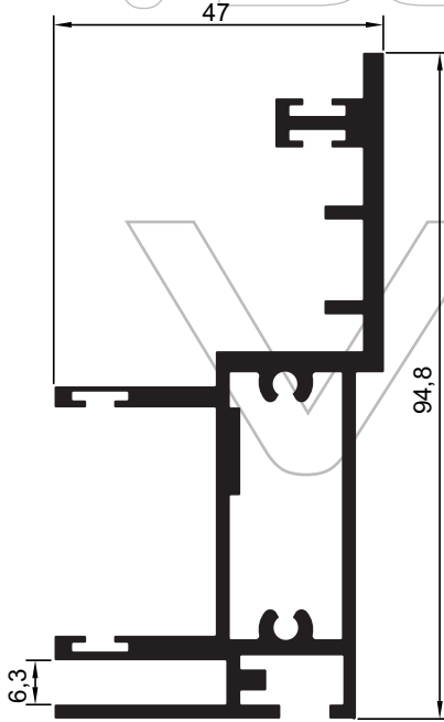
RK-102 Sabit Dikme 2.210 kg/m
