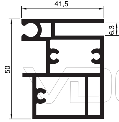
RK-104 Hareketli Yatay 1.580 kg/m
