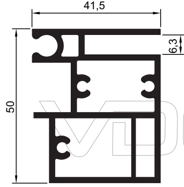
RK-104 Hareketli Dikme/Yatay 1.580 kg/m
