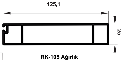
RK-105 Ağırlık 1.406 kg/m
