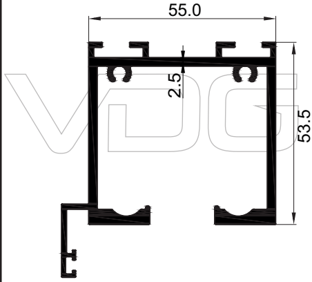
KK-101 Üst Kasa 1,750 kg/m
