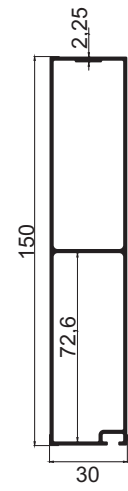
P-101 30x150 Kutu 1,711 kg/m
