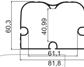
P-103 Kalın Korniş 1,280 kg/m
