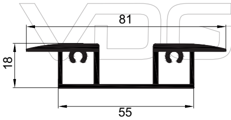
KK-104 Eşiksiz Alt Kasa 1,050 kg/m
