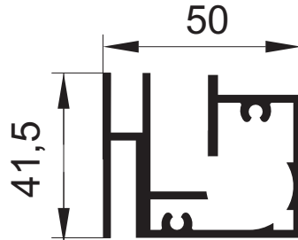
RK-106 Hareketli Çerçeve (Pistonlu) 1.592 kg/m
